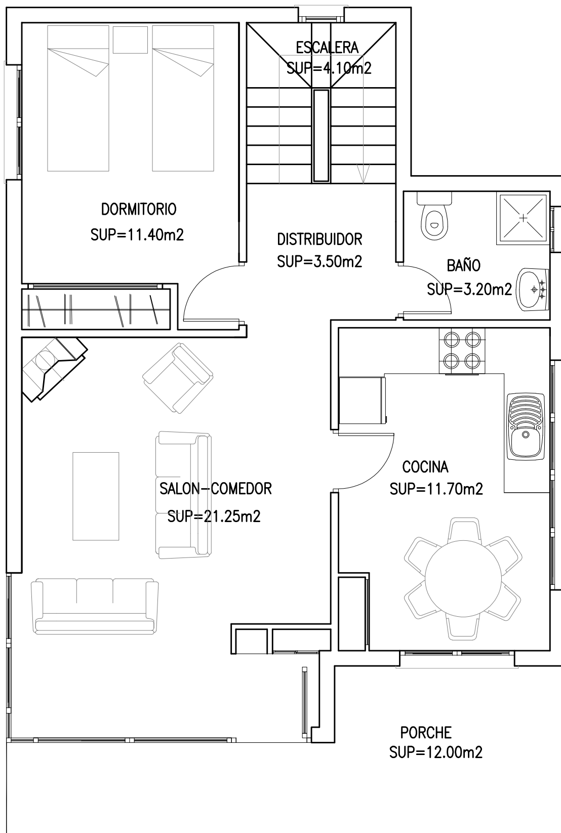
Planta Baja
